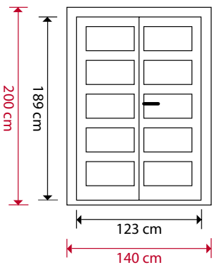
RC20 dubbele deur met matglas
