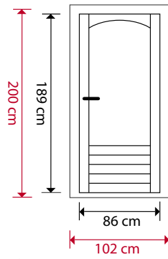
RC14 enkele deur met 75% glas
