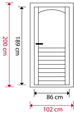
RC12 enkele deur met 50% glas
