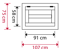
RC55 uitzetraam met matglas
