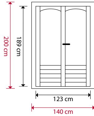
RC18 dubbele deur met 75% glas
