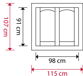
RC53 dubbel vleugelvenster
